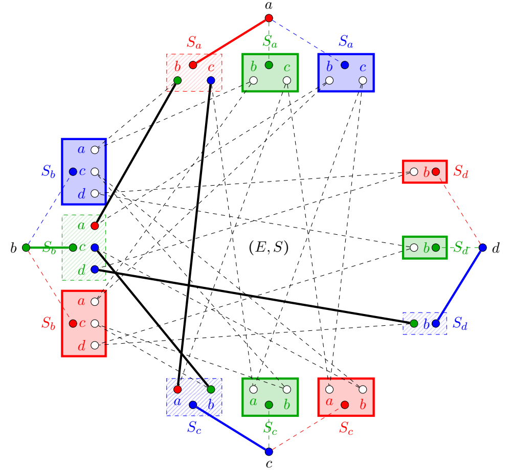
FIGURE 23. L'instance (E, S) associée au graphe G = (X, V) et la partition associée au 3-coloriage de la figure 22.
