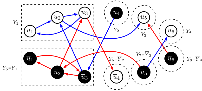
FIGURE 11. Graphe d'implication de (28) et ses 8 composantes fortement connexes.
