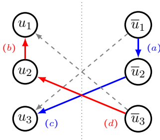
FIGURE 9. Graphe d'implication de (23) et sa fermeture transitive.
