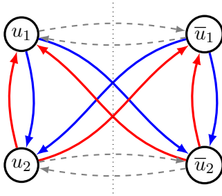
FIGURE 10. Graphe d'implication de (26) et sa fermeture transitive.
