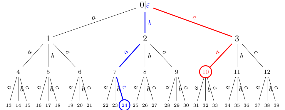
FIGURE 2. Les 4 premiers niveaux de l'arbre lexicographique du langage \{a, b, c\}^* et l'indexation des mots.
