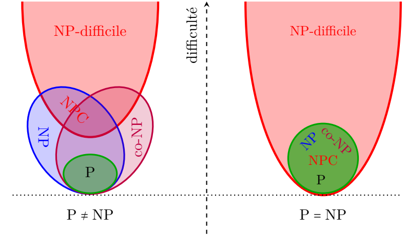
FIGURE 5. Hiérarchies simplifiées des classes de complexité selon la validité de la conjecture.
