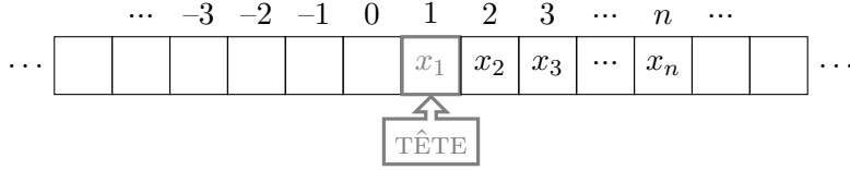
FIGURE 3. Schématisation d'une machine de Turing.
